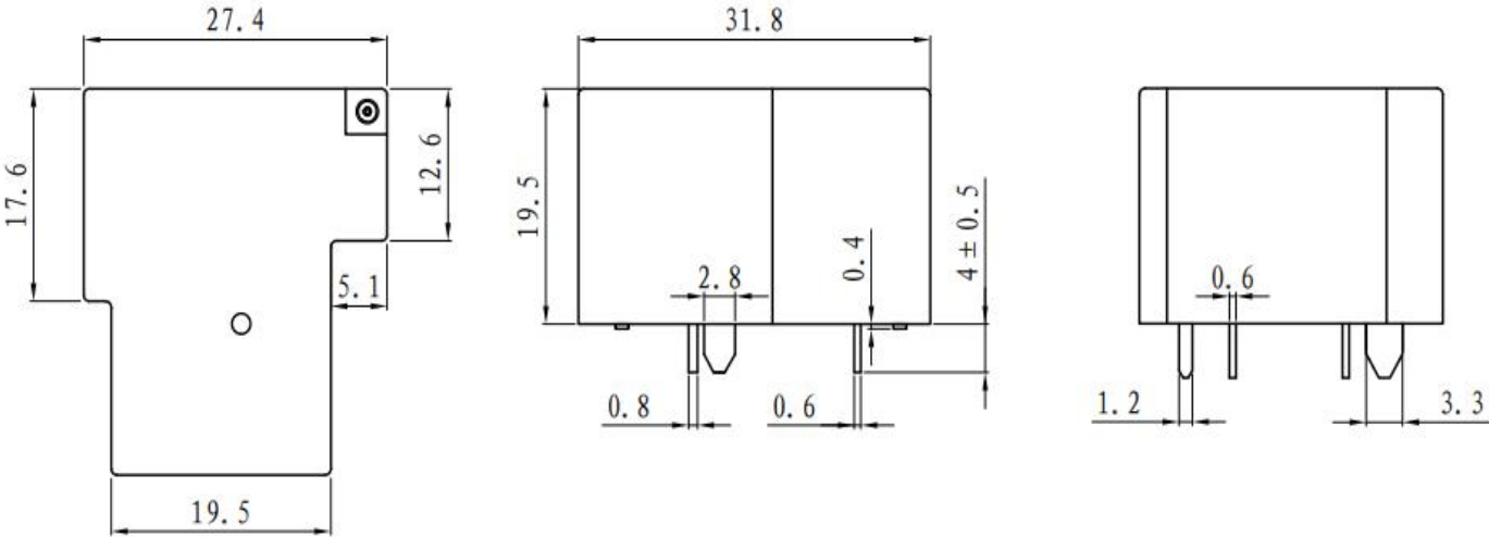
外形尺寸 Outline Dimensions
